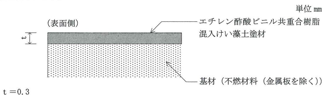
図 1 断面図
